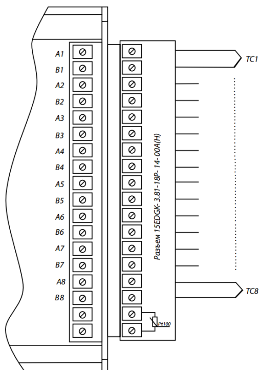
Рисунок 1.3 – Схема подключения термодпар
